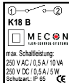
Fig. 8 Contact K 18 B
